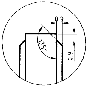
Detaliu A (5:1)
